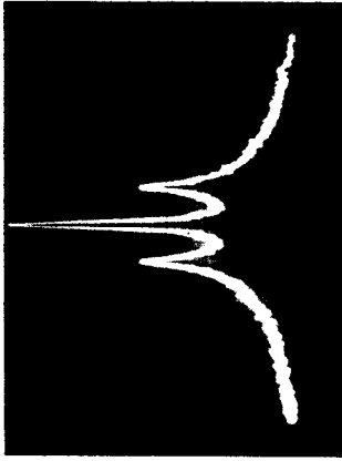
9A. Horizontal - 20 kHz/Div. Vertical - 10 dB/Div. Center - 8.0 GHz
